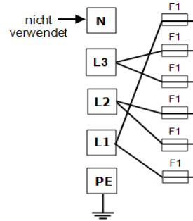
Dreieckschaltung
