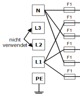
Einphasenschaltung
